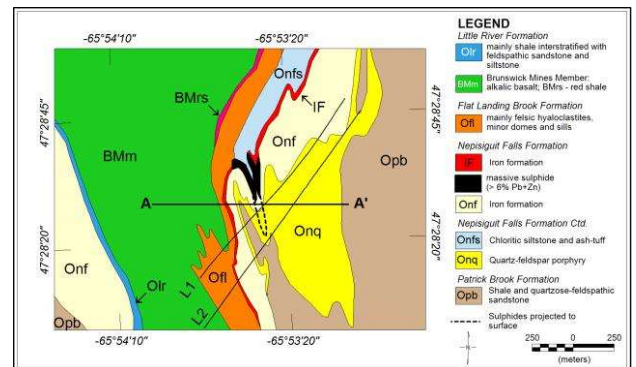
Fig. 1 – Mapa geológico simplificado da região de Brunswick No. 12 (Thomas et al., 2000).
