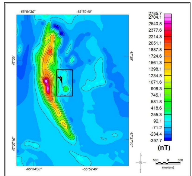
Fig. 2 – Campo magnético residual da região de Brunswick No. 12. O retângulo preto localiza a região omitida para a reinterpolação.
